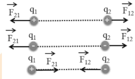
Hình 2.1: Lực tương tác giữa 2 điện tích
